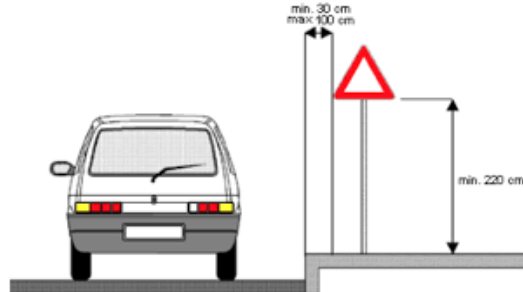
INSTALLAZIONE A LATO CARREGGIATA
